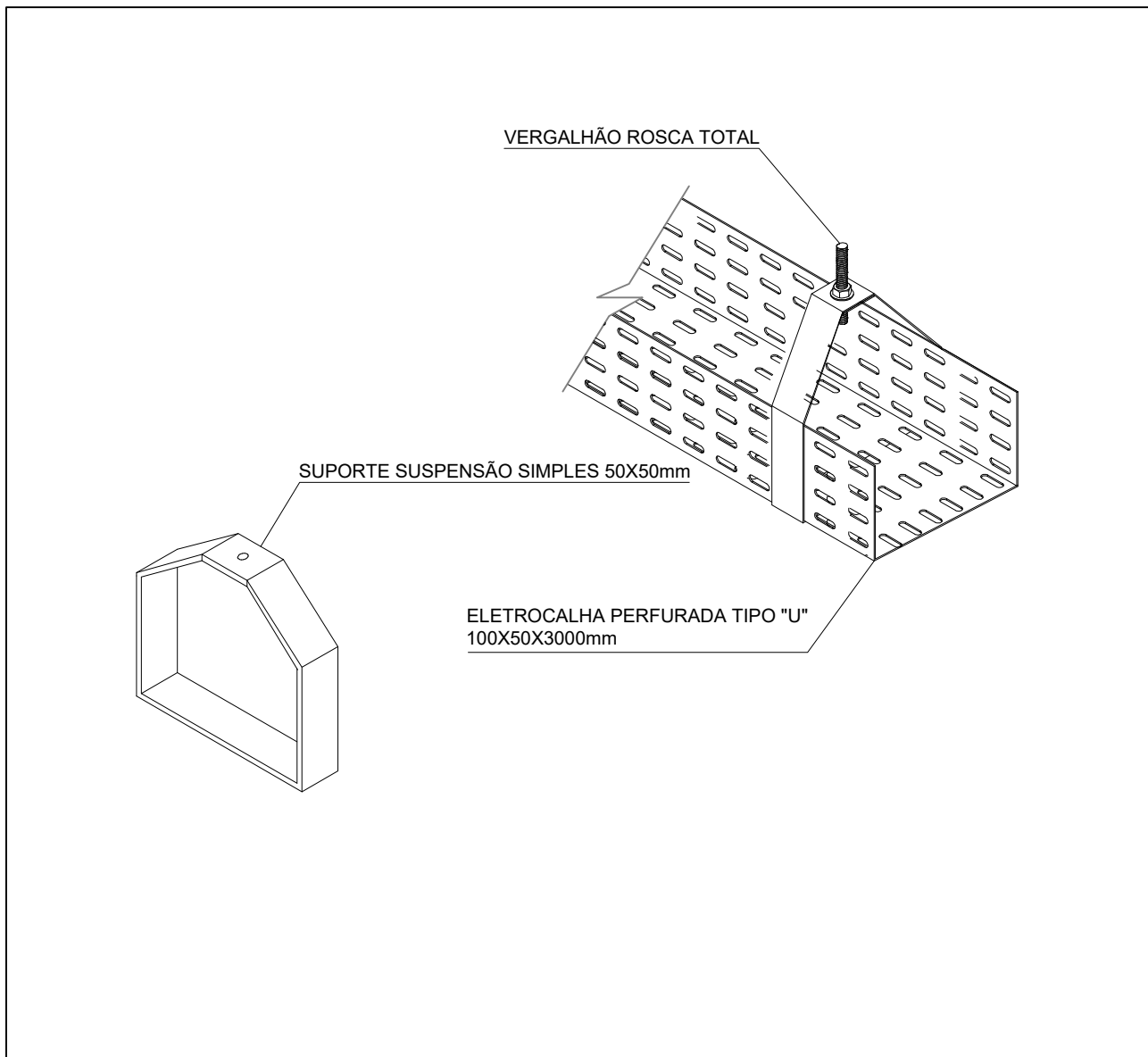
DETALHE 2: SUPORTE PARA ELETROCALHA ESCALA: S/N
