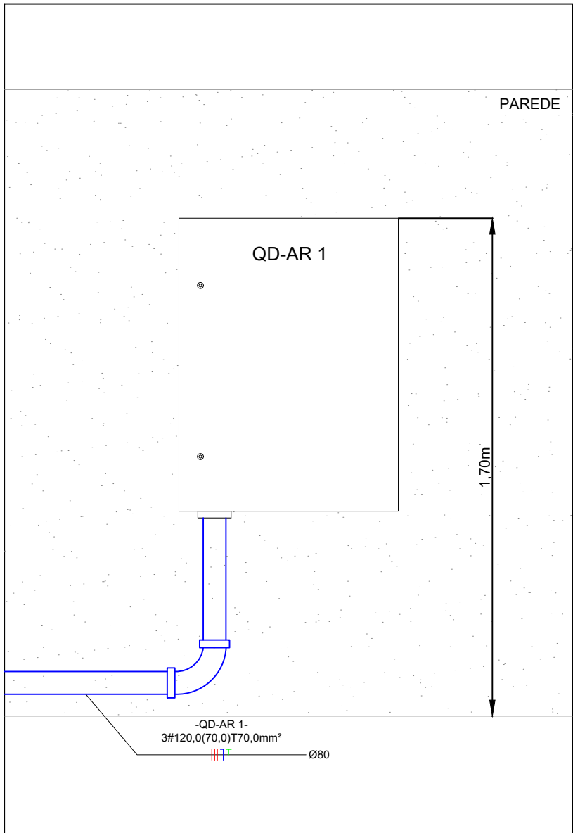
DETALHE 3: VISTA FRONTAL DO QD-AR 1 ESCALA: S/N
