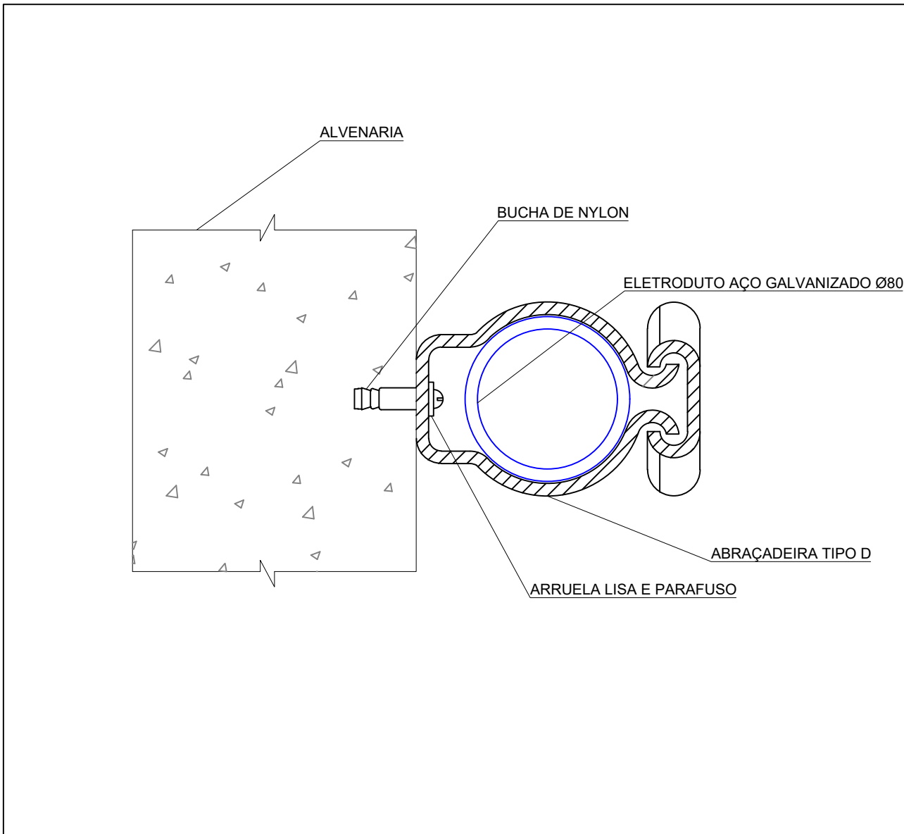
DETALHE 1: SUPORTE PARA ELETRODUTO ESCALA: S/N
