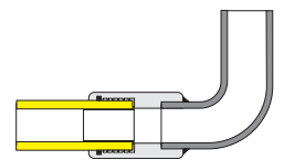
Transição de Afloramento Metal-PE Tipo Riser
