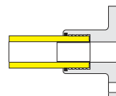
Transição Metal-PE Flangeada Tipo F
