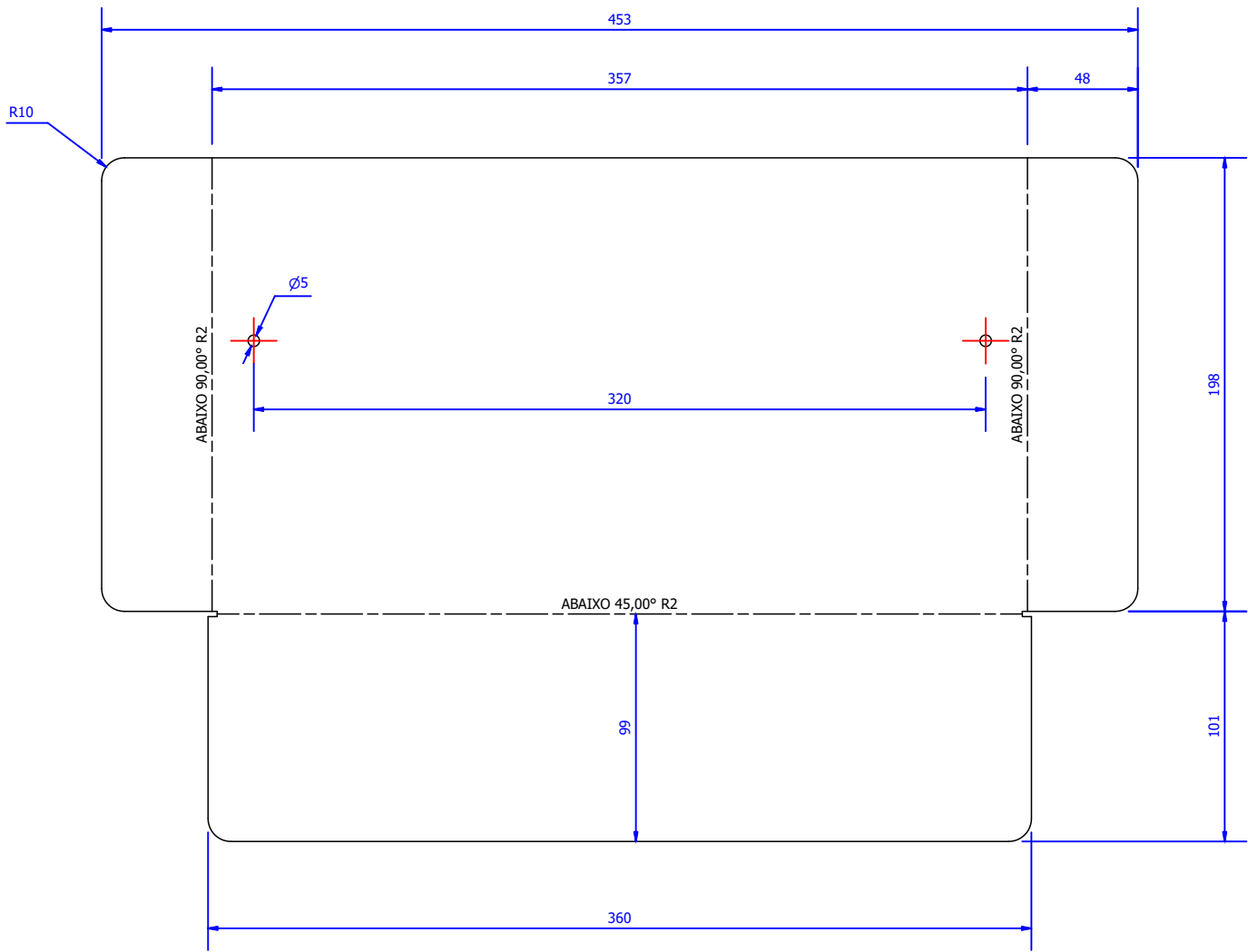
DETALHE DA CHAPA ( 1 : 3 )
