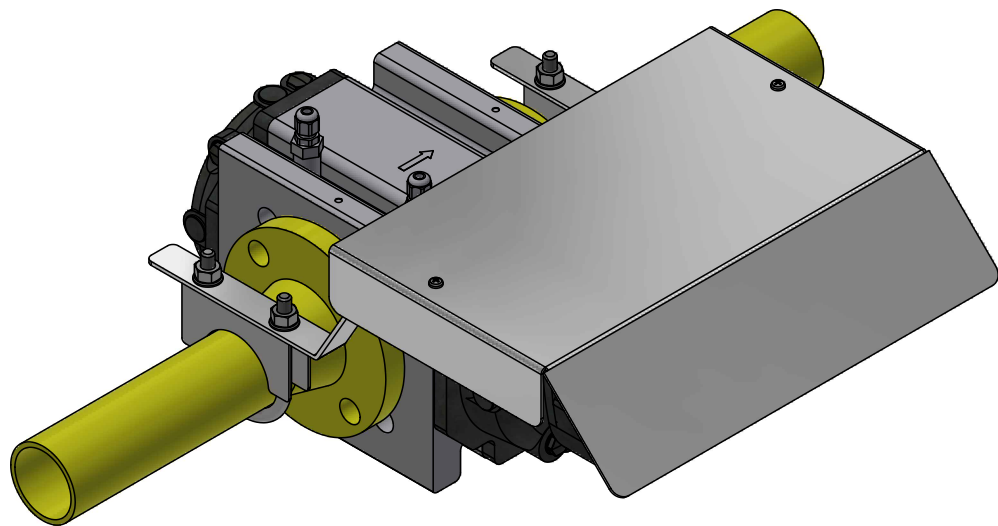
PERSPECTIVA ( 1:5 )
