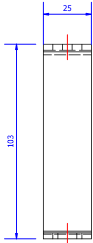
VISTA LATERAL ESQUERDA ( 1 : 2 )
