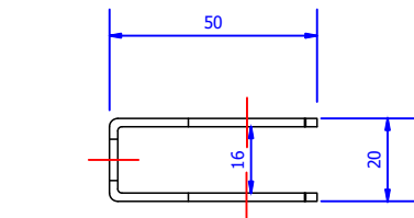
VISTA FRONTAL ( 1 : 2 )
