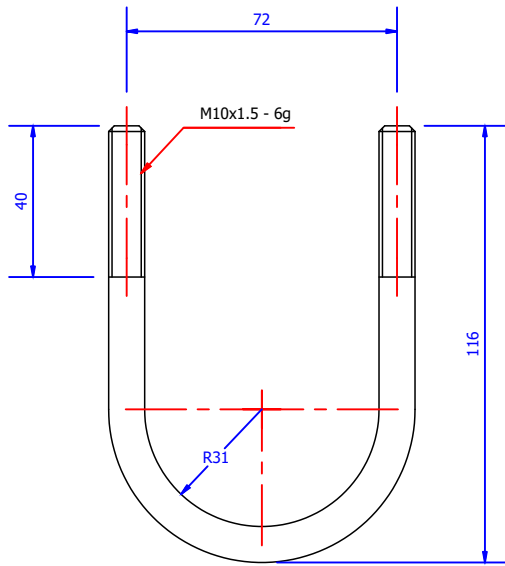
DETALHE GRAMPO ( 1 : 2 )
