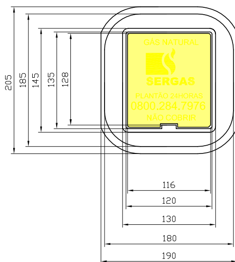
VISTA SUPERIOR
