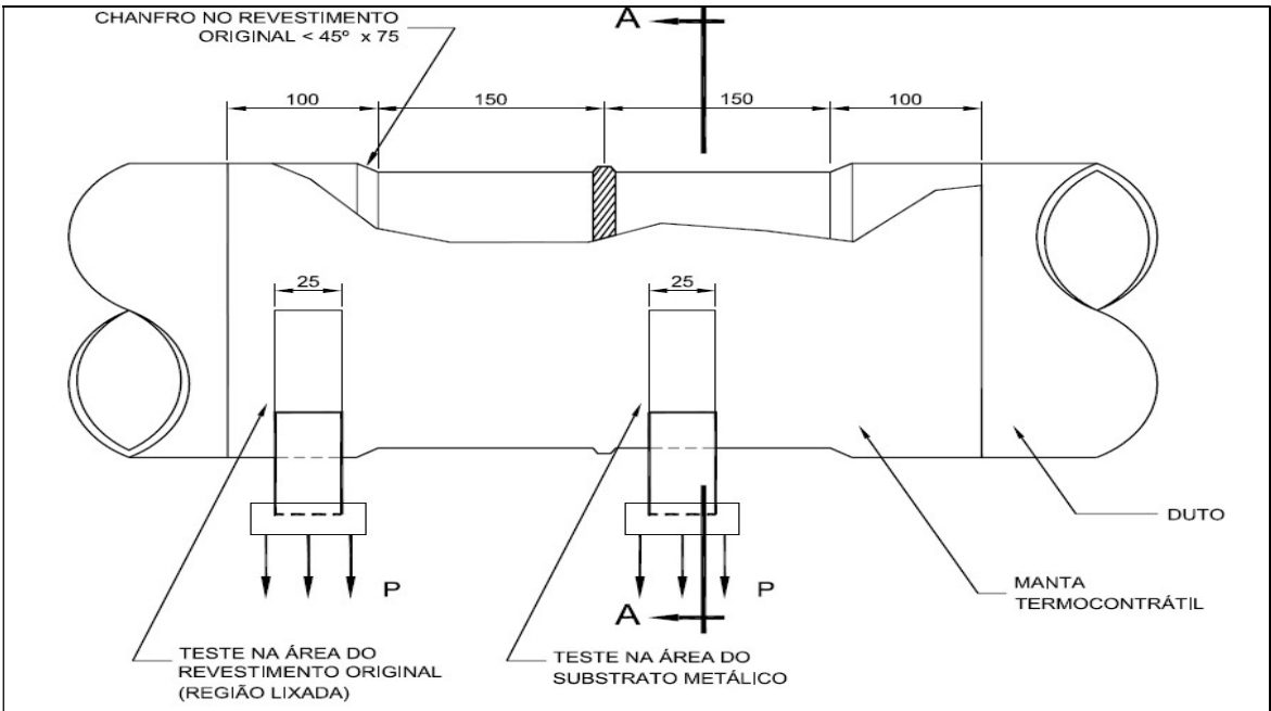
Figura 26: Teste de aderência de fita anticorrosiva.
